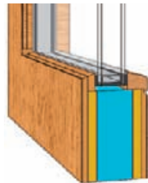
C letvica znotraj zamik stekla 22 mm na zunanji strani
